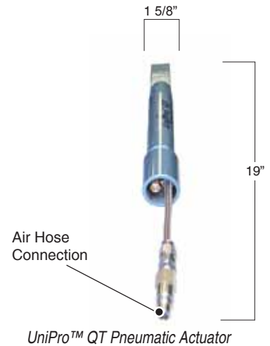
UniPro™ QT Pneumatic Actuator
